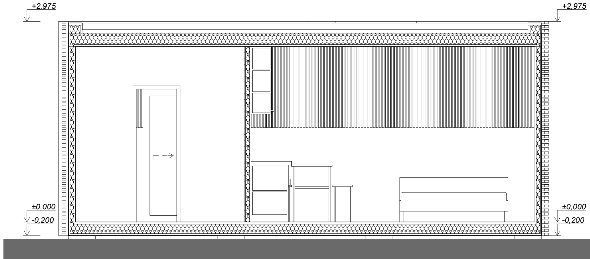
ŘEZ PODÉLNÝ
