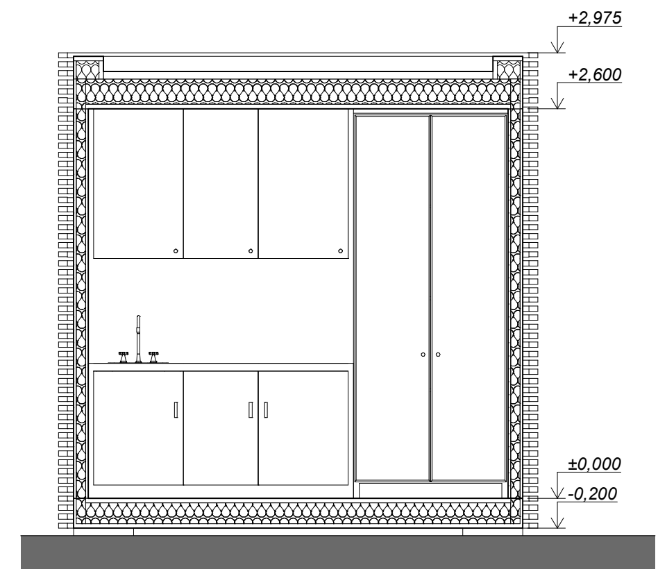
ŘEZ PŘÍČNÝ
