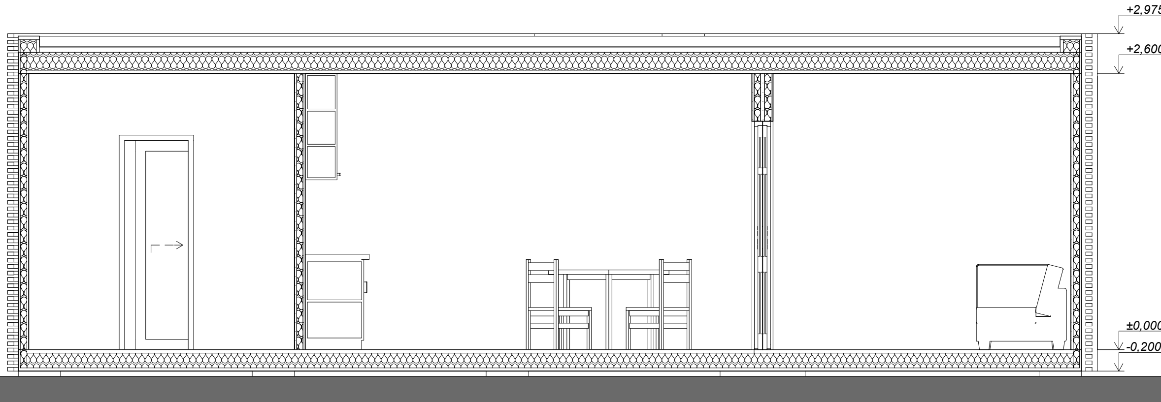
ŘEZ PODÉLNÝ
