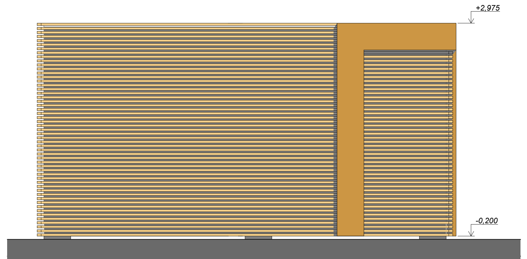
POHLED BOČNÍ
